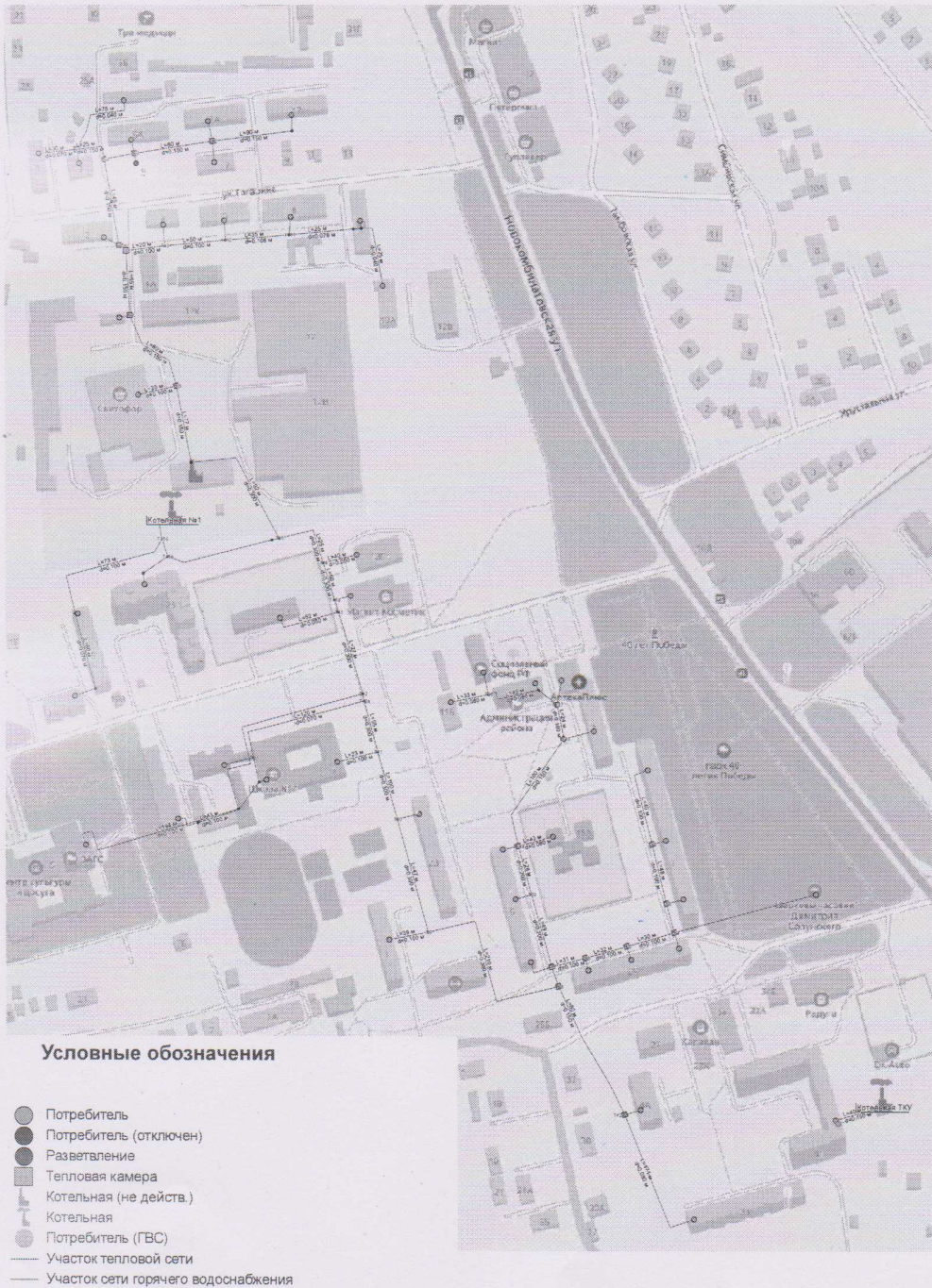
Приложение 2 - Схема теплоснабжения р.п. Ишеевка (Котельная №1, Котельная ТКУ 2000В)
