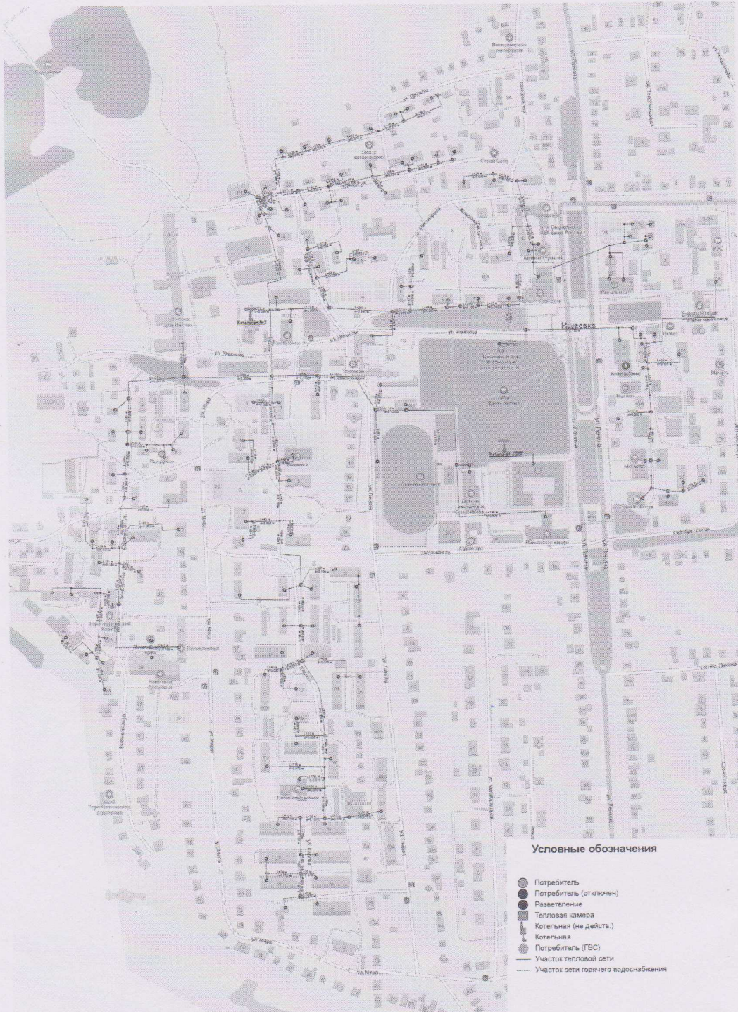
Приложение 1 - Схема теплоснабжения р.п. Ишеевка (Котельная №2, Котельная СОШ)
